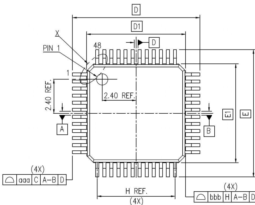
图 26 LQFP48 封装图
