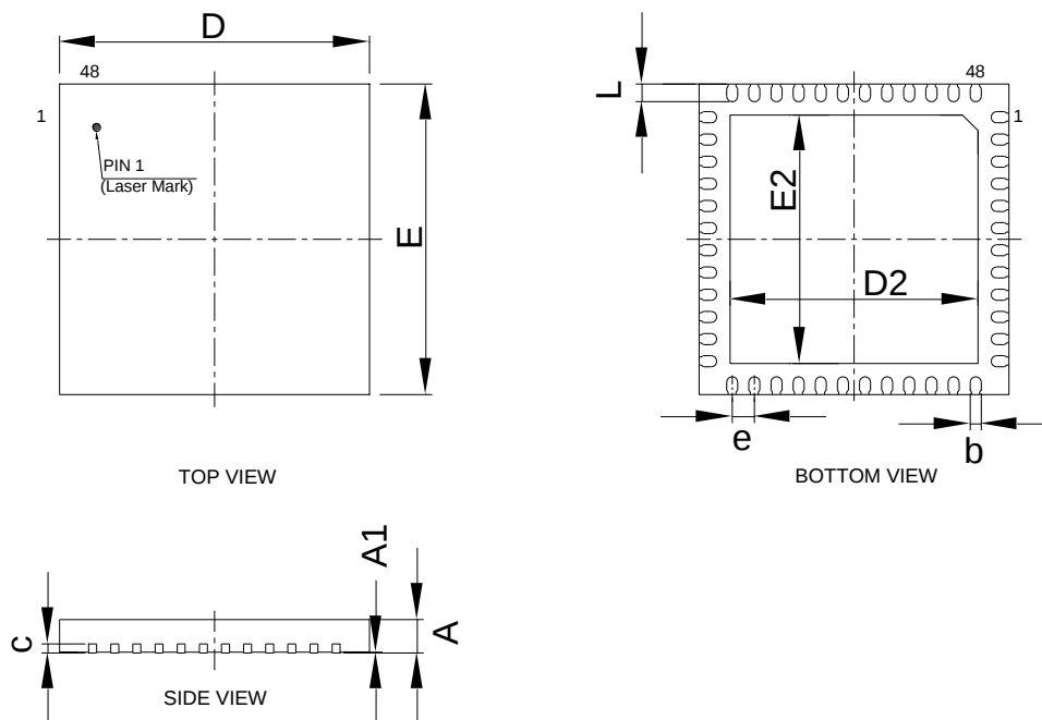
图 29 QFN48 封装图
