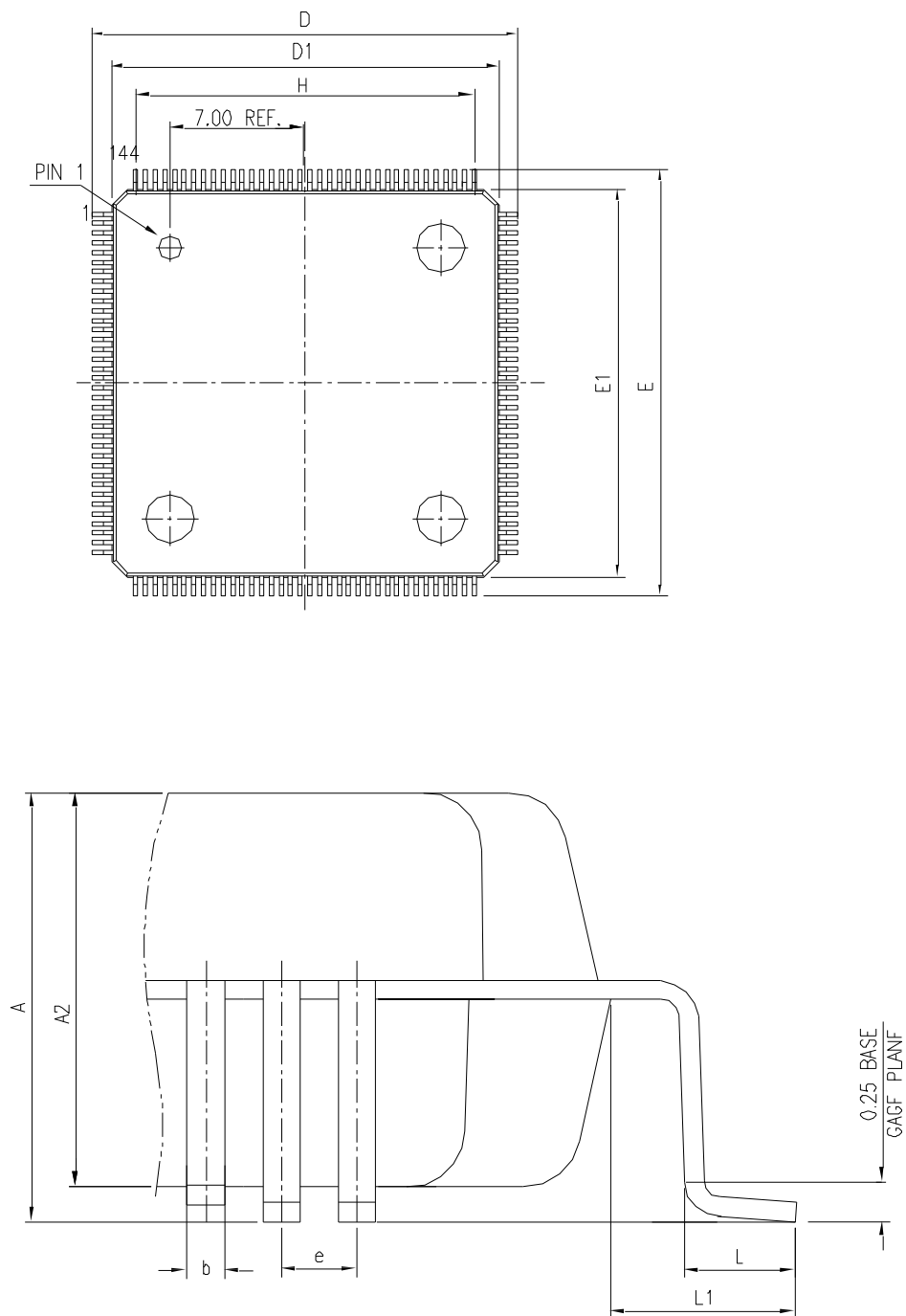
图 17 LQFP144 封装图
