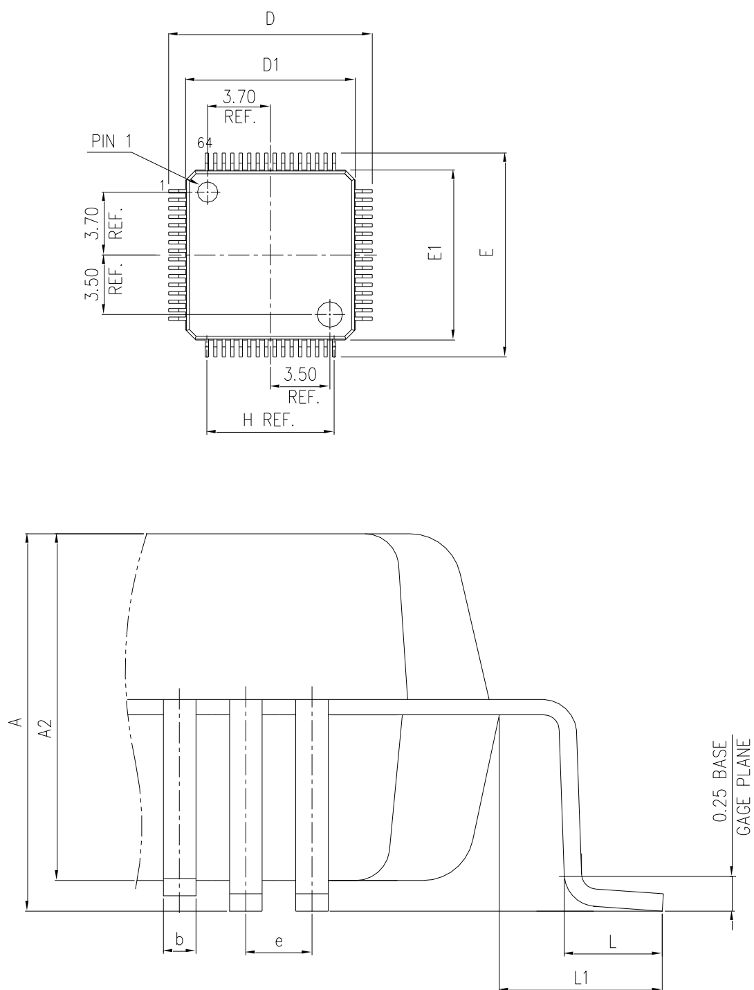
图 23 LQFP64 封装图
