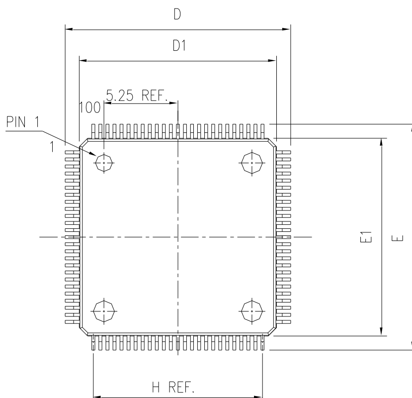
图 20 LQFP100 封装图
