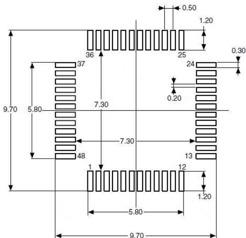
图 27 LQFP48, 7×7mm 焊接 Layout 建议
