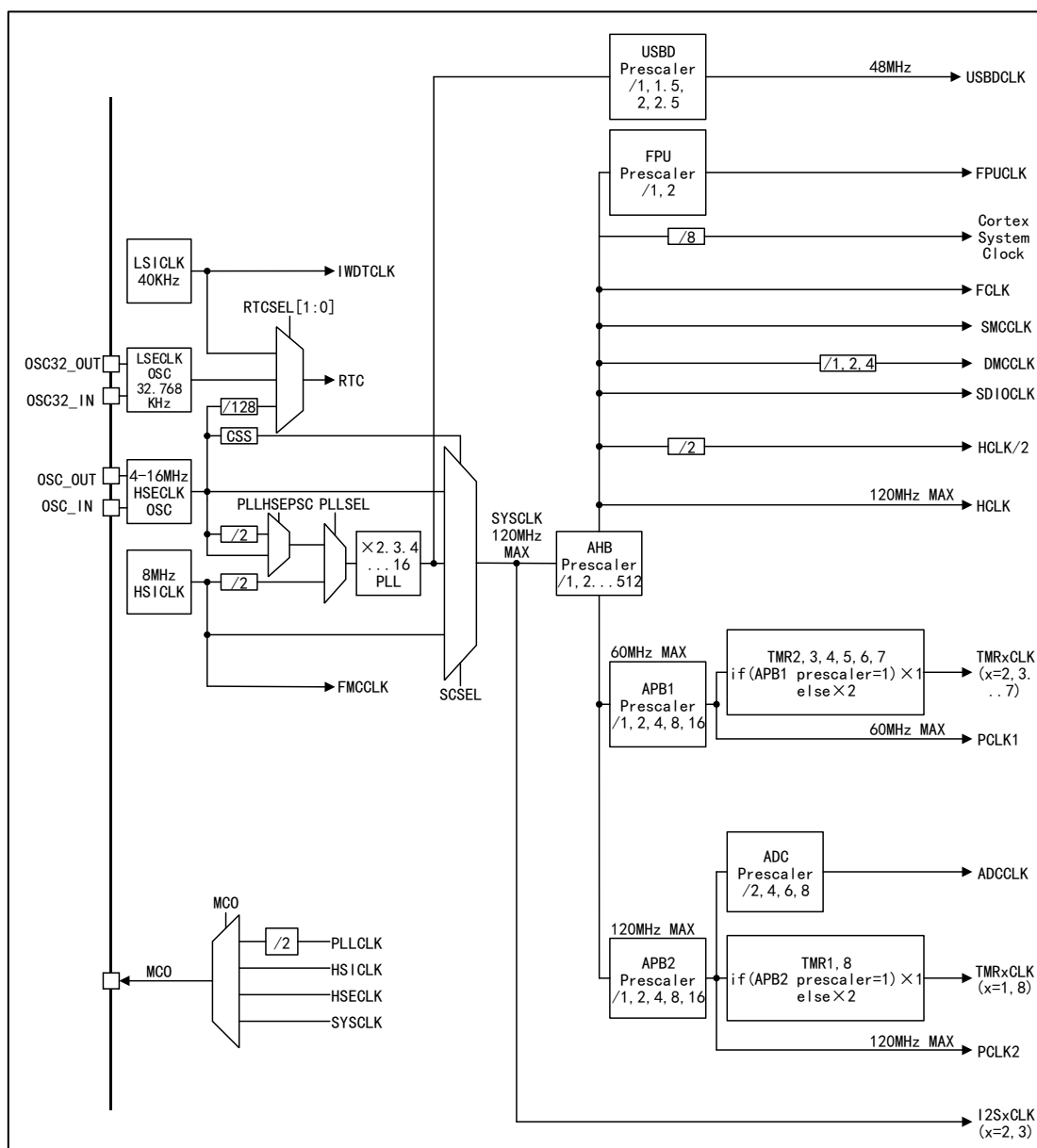
图 7 APM32E103xCxE 时钟树
